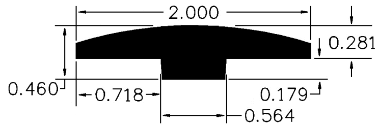
T-Molding (HTMLD)
